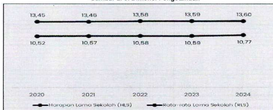
Gambar 2. 5. Dimensi Pengetahuan
